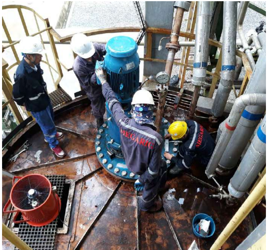
Sửa chữa bảo dưỡng, cân bằng động cánh bơm nhà máy ANP Thái Bình/ Repairing, maintain, and balance pump impellers of Thai Binh ANP factory
