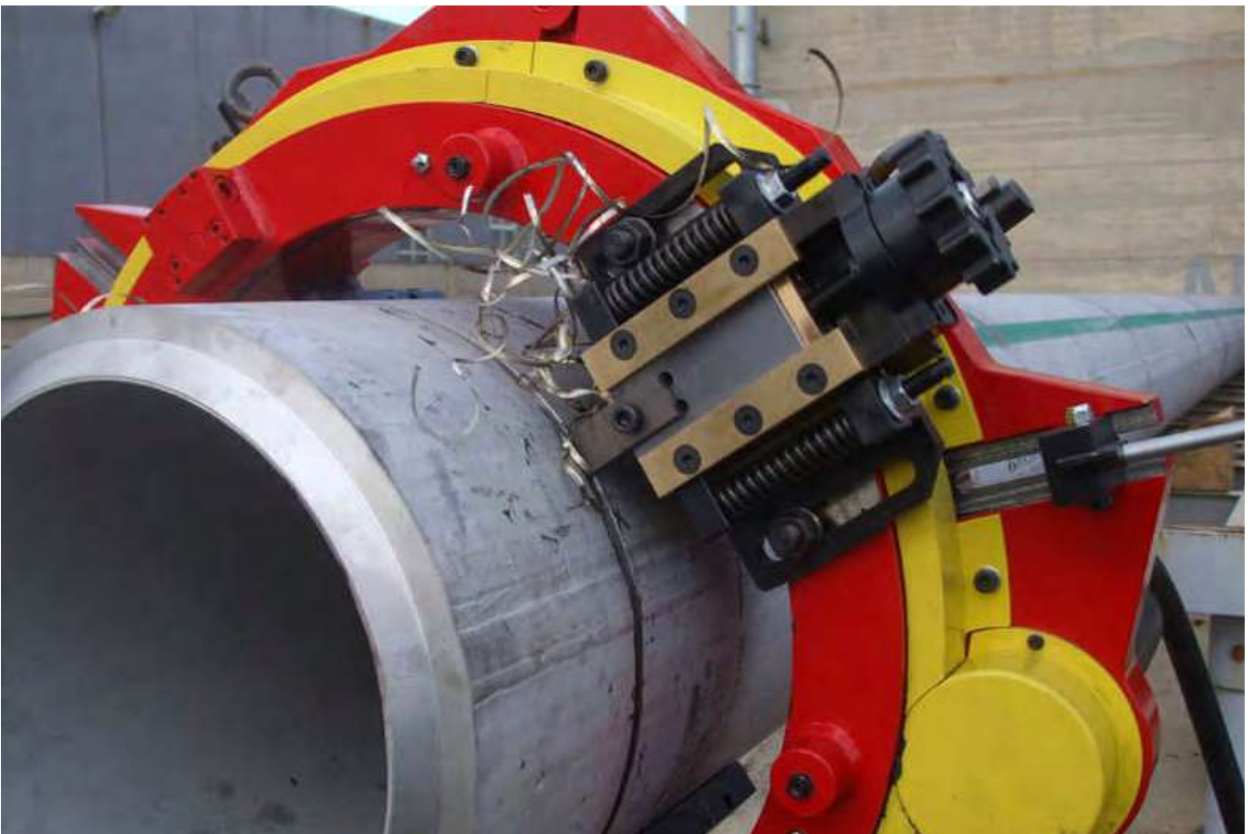
Cắt và vát mép ống bằng phương pháp cắt nguội/Pipe cold cutting & Pipe beveling.
