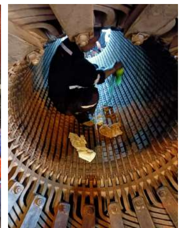
Thi công sửa chữa Tuabin Nhà máy Nhiệt Điện Nông Sơn / Construction and repair of turbines for Nong Son Thermal Power Plant
