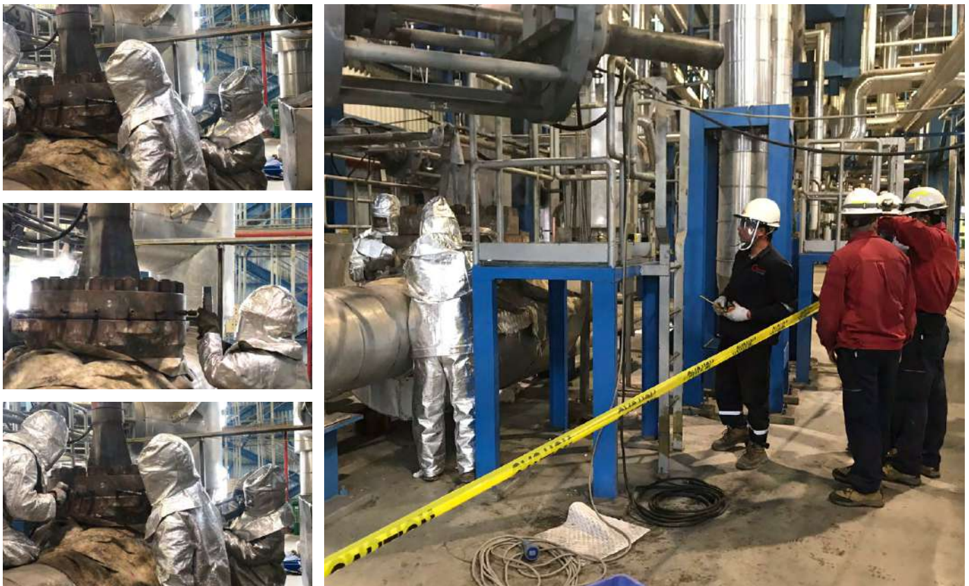
Sửa chữa rò rỉ của van điều khiển đường ống Nhà máy nhiệt điện Mông Dương 2/ Repair leaks of pipeline control valves in Mong Duong 2 Thermal Power Plant
