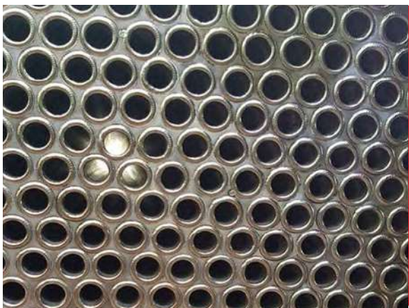
Hoàn thiện công tác thay thế ống Tube/Finishing re-tube work
